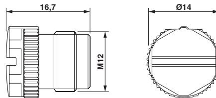
Målskisse
