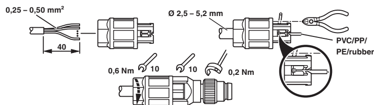
Funksjonstegning
