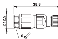
Målskisse
