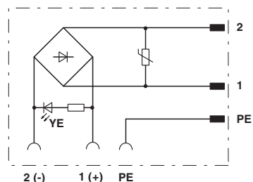
Koblingskjema
