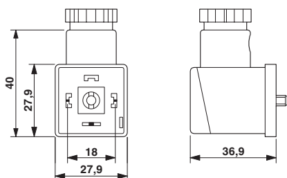
Målskisse
