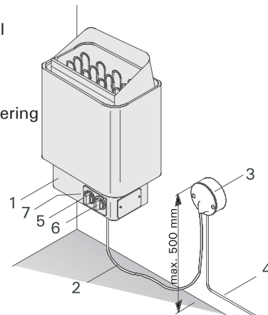
Skisse 1. Komponenter og tilkopling av ovn. Iflg. den til enhver tid gjeldende NEK400-norm kan tilkoplingskabel føres direkte inn i ovn.
