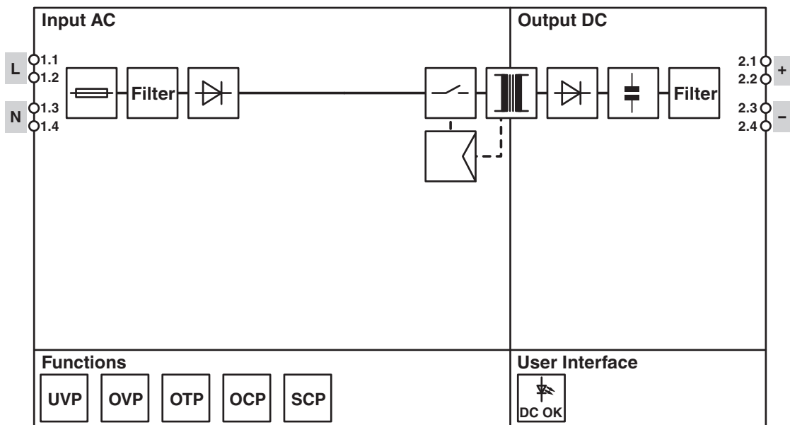
Blokkskjema
