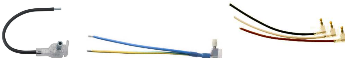
KF50B Overgangskabel al-cu 50/16mm, KF50E PE-N Overgangskabel al-cu 50/16mm 2 , KF50H 3xOvergangskabel al-cu 50/16mm 2
