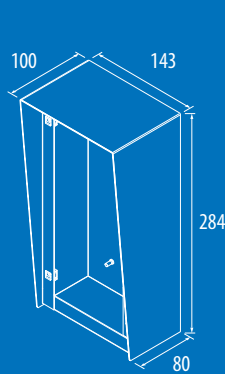
VRDSB140x280
