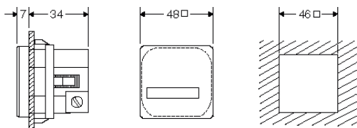
Frontramme 48 x 48 mm. Montering med festebøyle.
