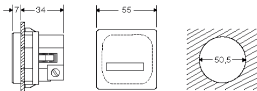
Frontplate med ramme 55 x 55 mm. Montering med festebøyle.
