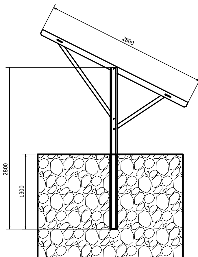
Rys.1 Wymiary konstrukcji
