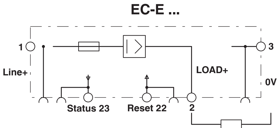
Koblingsskjema
