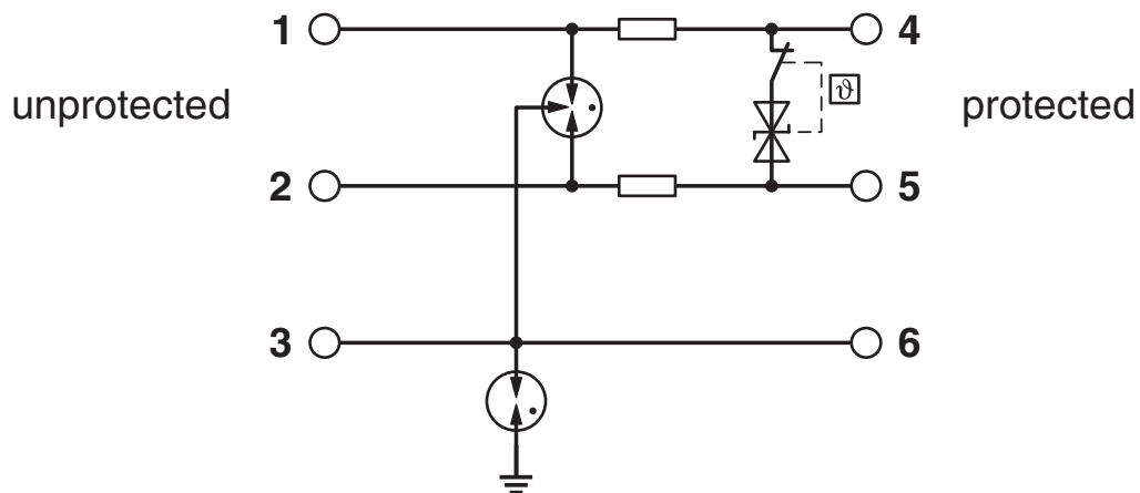
Koblingsskjema
