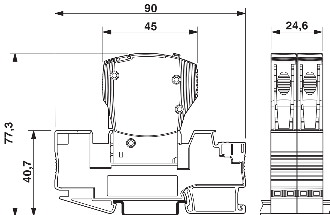
Målskisse
