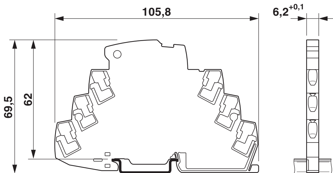
Målskisse
