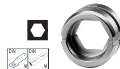
Bakk for press av DIN-normerte kabelsko og skjøtehytter Al
