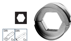
Bakk for press av DIN-normerte kabelsko og skjøtehytter Cu
