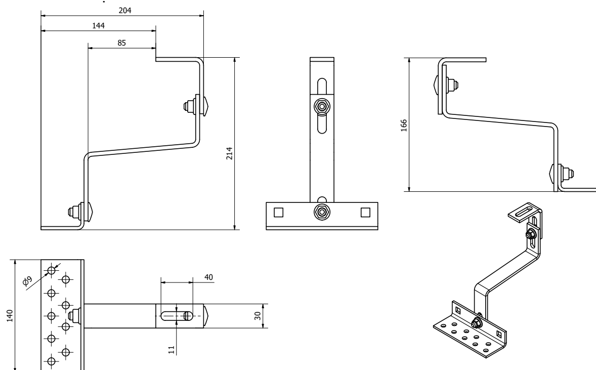
Fig. 3 K-12+3 Element dimensions
