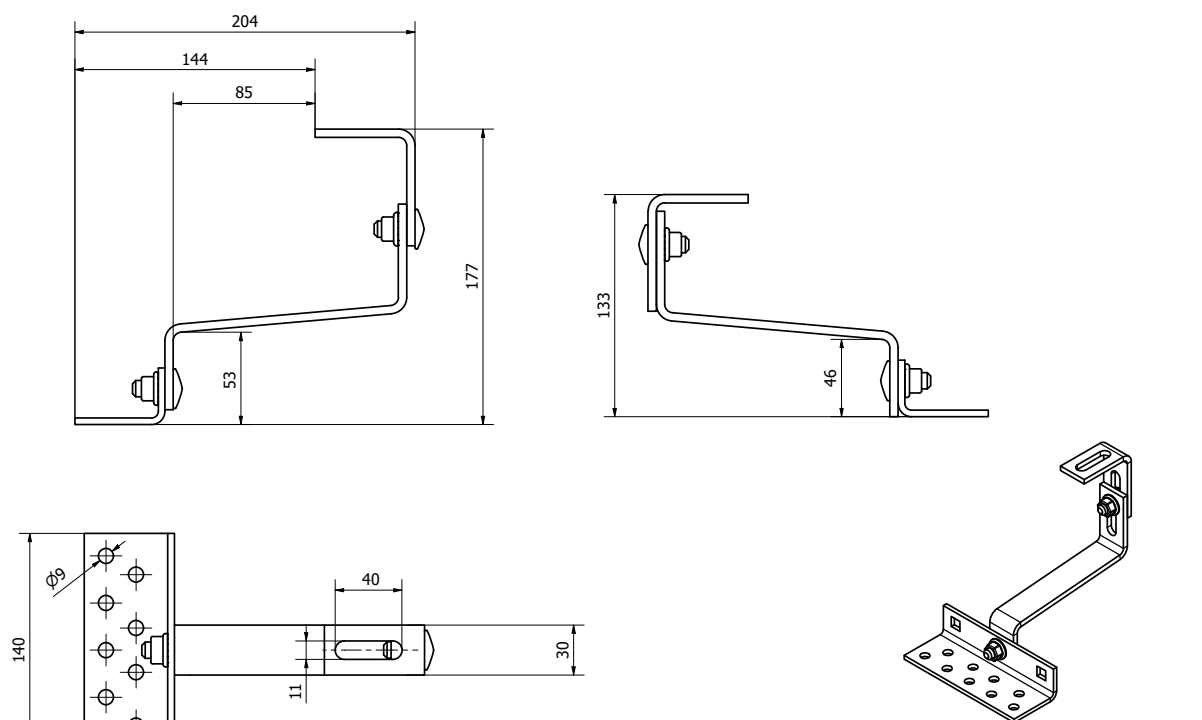
FIG1 K-12 Element dimensions
