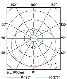
Light Distribution Diagram - CorePro LEDtube UN 1500mm UO 23W865 T8
