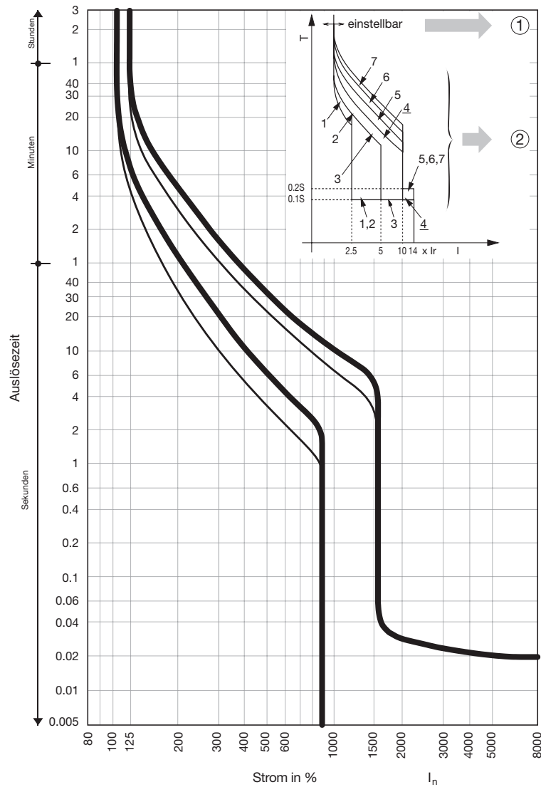
Zeit-Strom-Kennlinie HNF, HEF, 3-/4-polig
