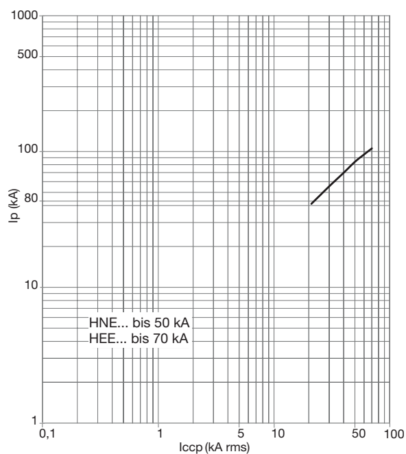
Kurzschlussstrom-Bergrenzungskennlinie ( I_p ) HNF, HEF, 3-/4-polig
