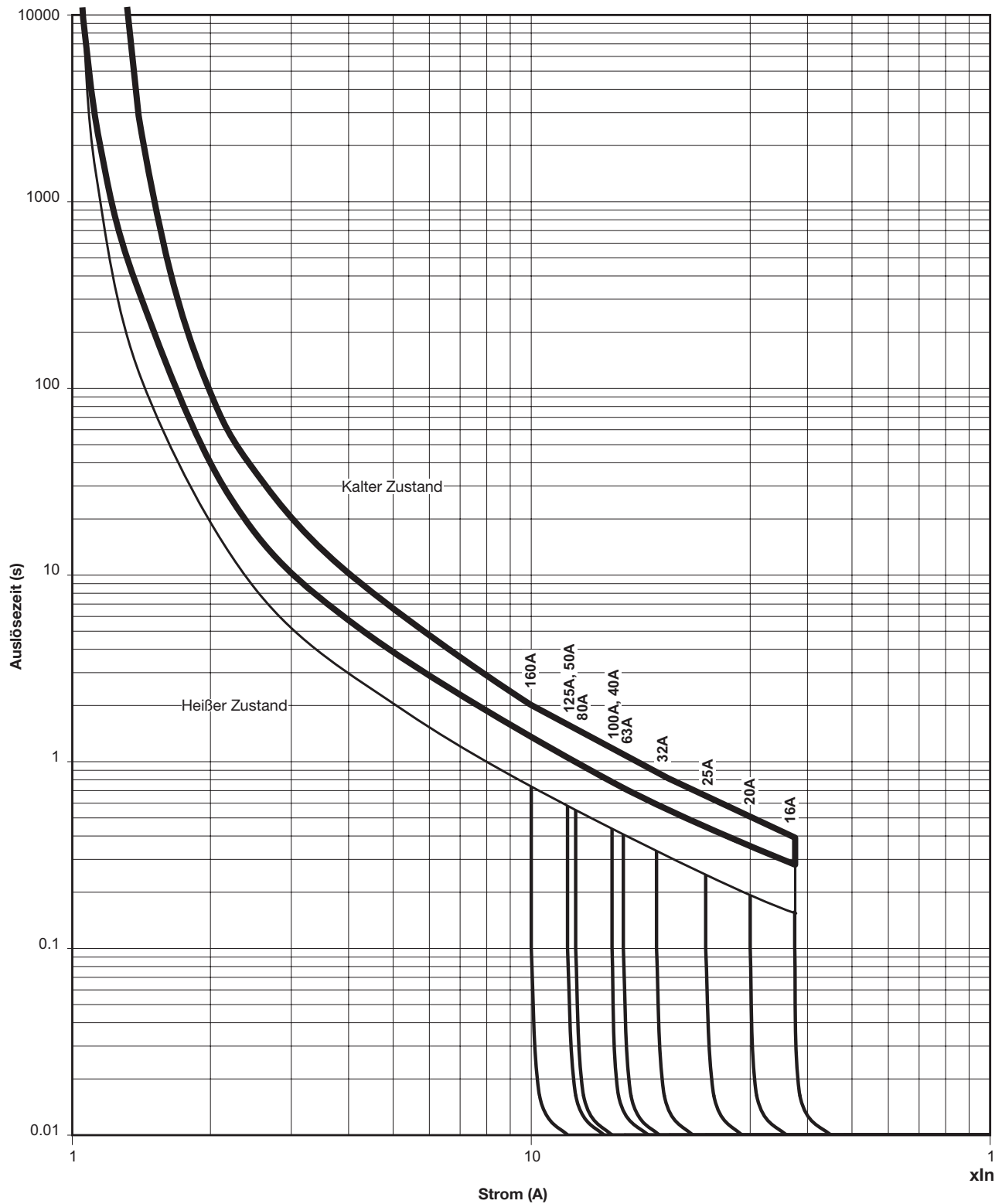
Zeit-Strom-Kennlinie
