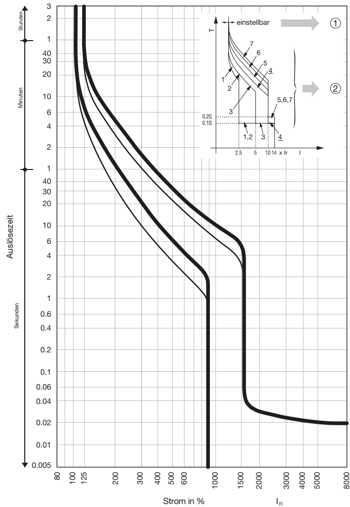
Zeit-Strom-Kennlinie für Leistungsschalter 1000 A HNE, HEE, 3-/4-polig
