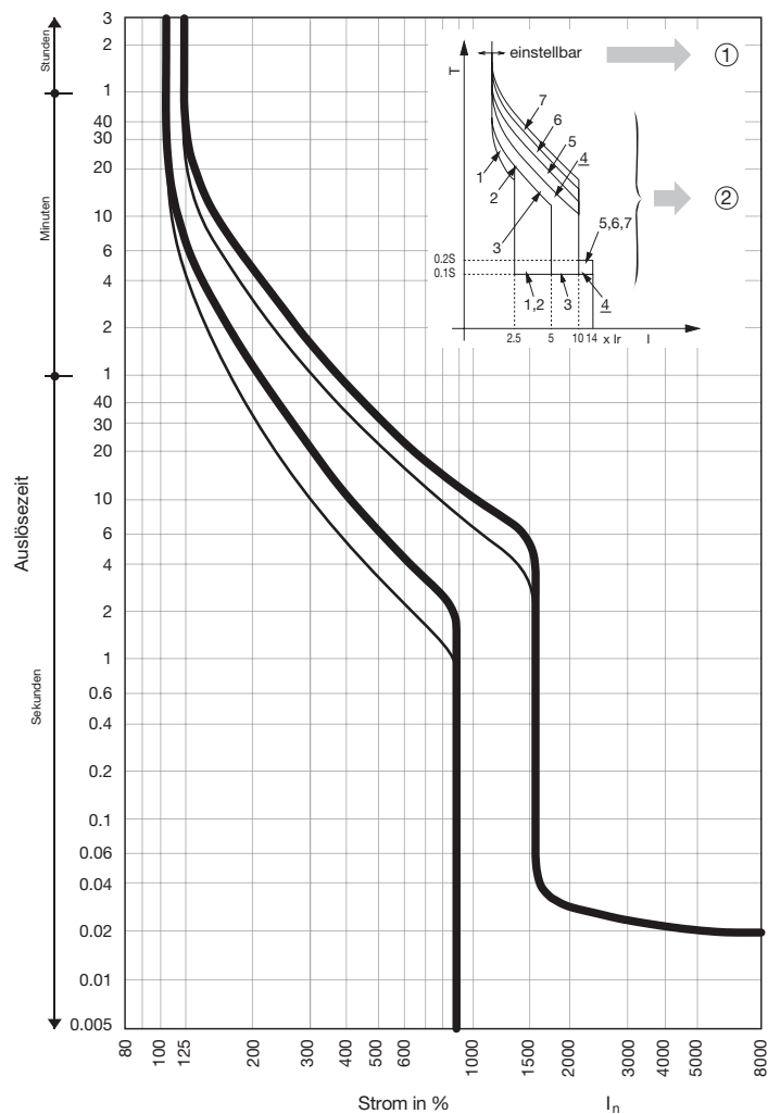
Zeit-Strom-Kennlinie für Leistungsschalter 800 A HNE, HEE, 3-/4-polig
