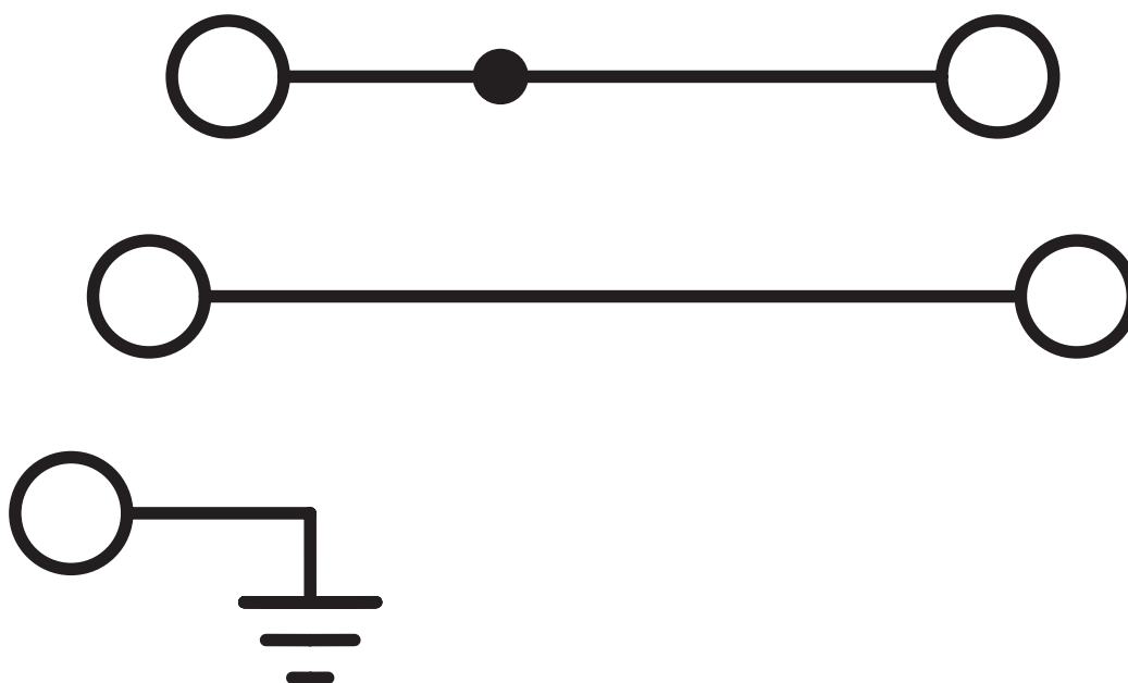
Koblingsskjema
