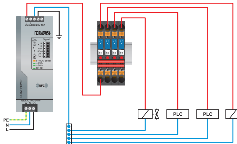
Applikasjonstegning
