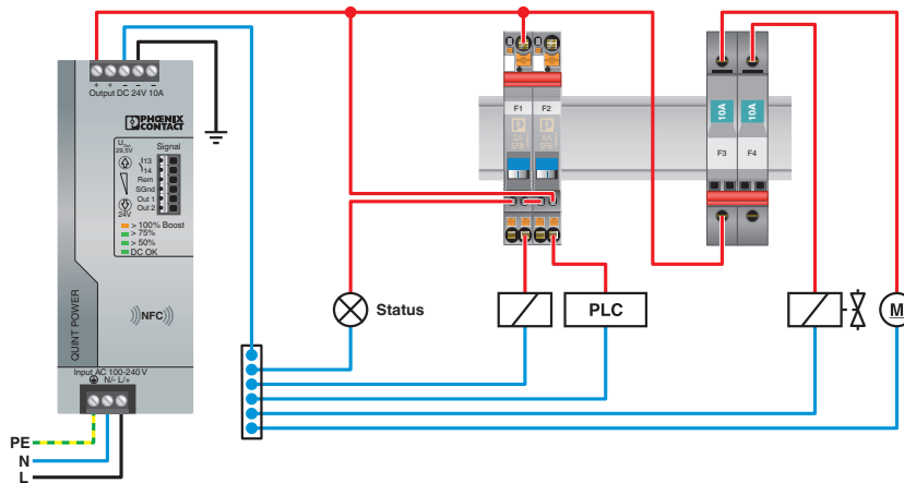
Applikasjonstegning
