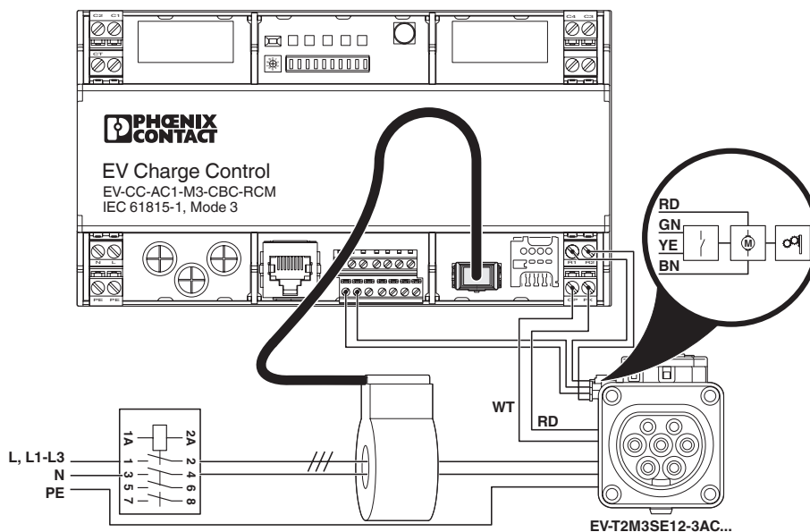
Tilkoblingstegning
