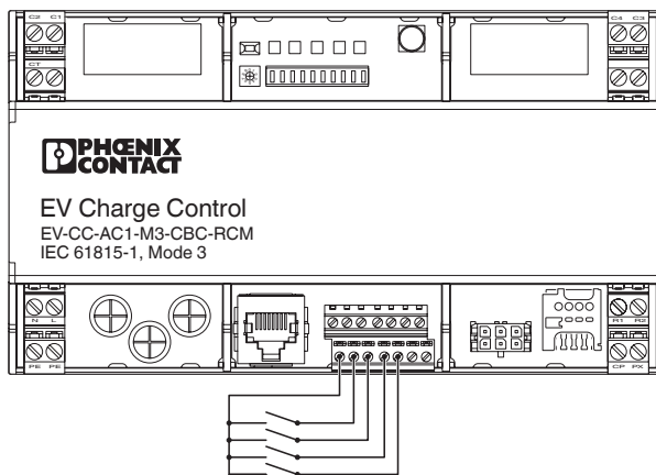
Tilkoblingstegning
