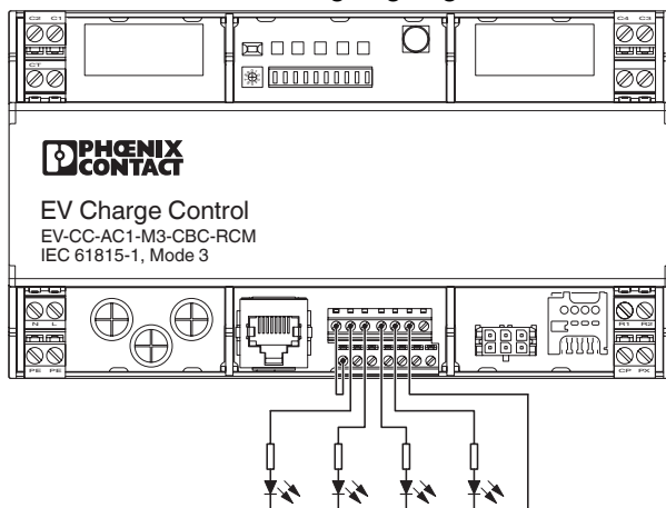
Tilkoblingstegning
