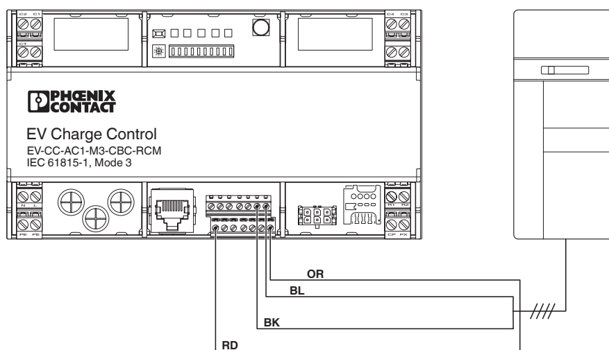
Tilkoblingstegning
