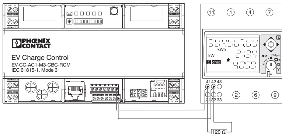
Tilkoblingstegning
