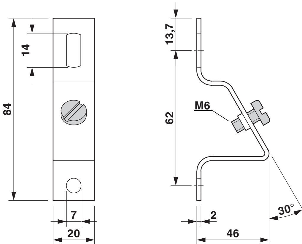
Målskisse
