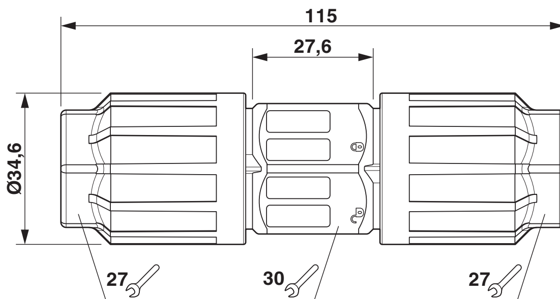
Målskisse QPD C 5x2,5
