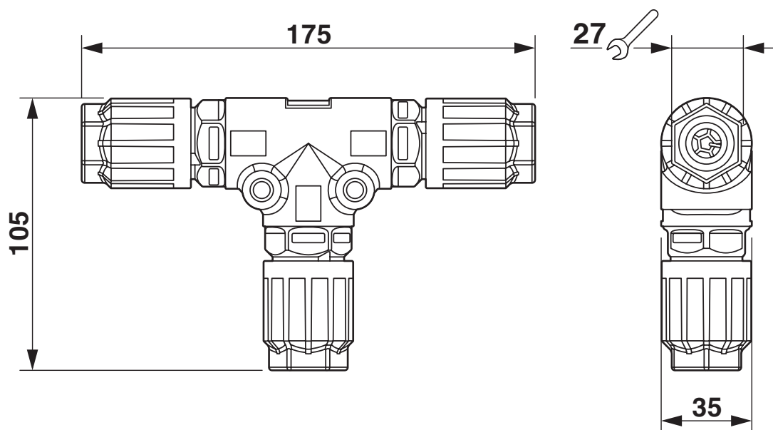
Målskisse
