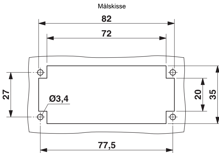
Monteringsåpning ved bruk uten hus
