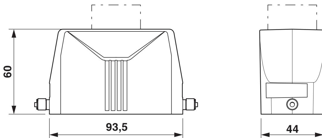
Målskisse
