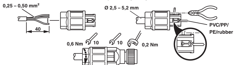
Funksjonstegning
