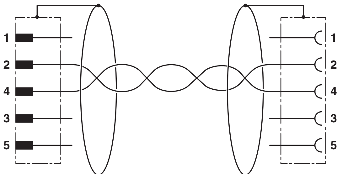
Koblingsskjema
