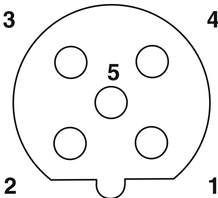
Skjemategning
