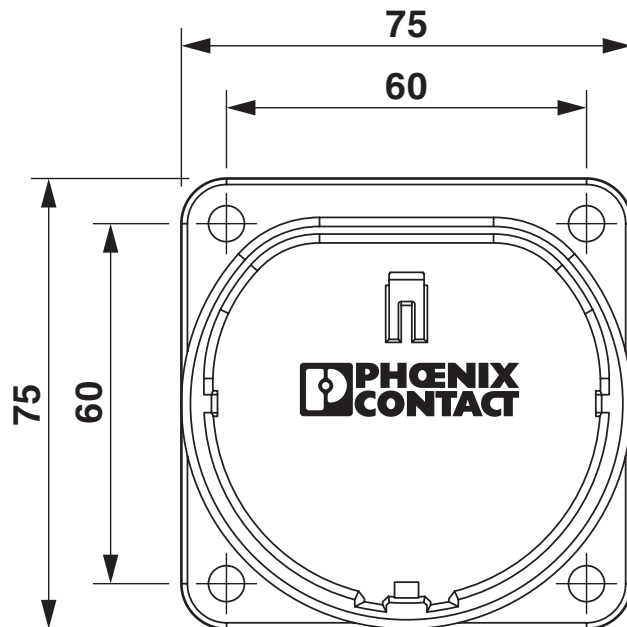
Målskisse
