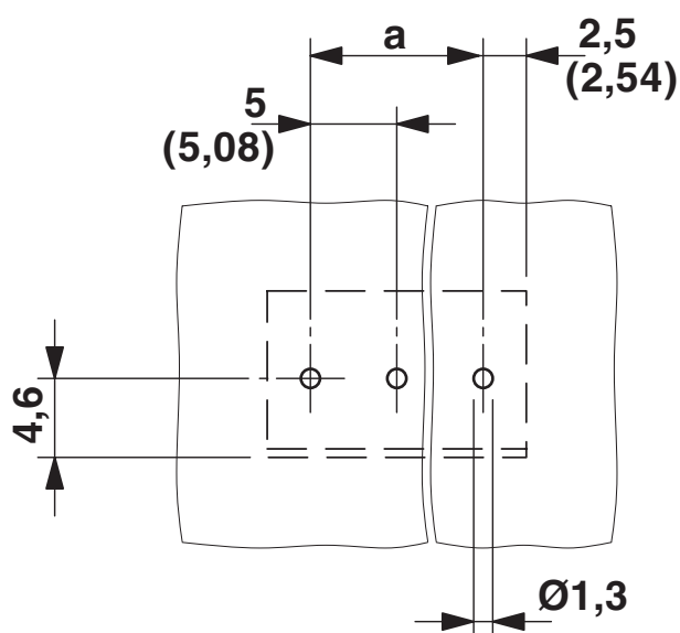
Boreplan/loddeputegeometri
