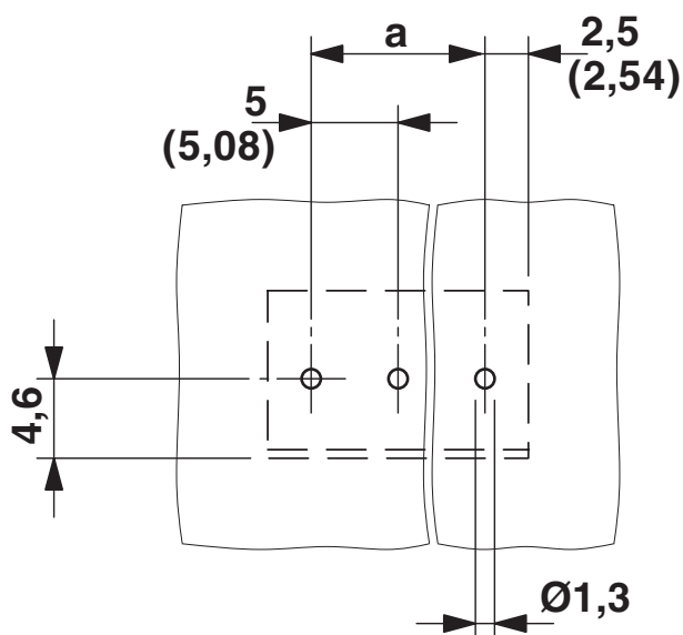
Boreplan/loddeputegeometri
