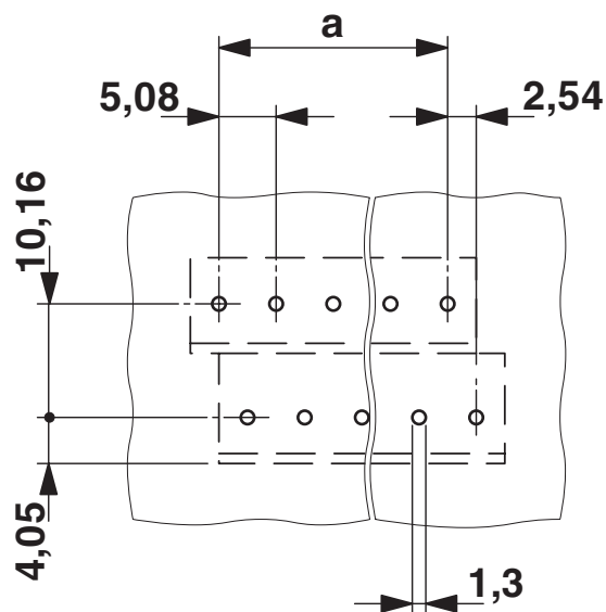
Boreplan/loddeputegeometri
