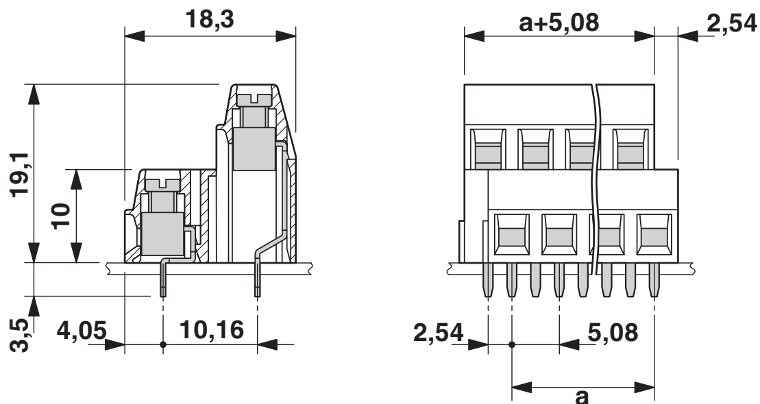
Målskisse
