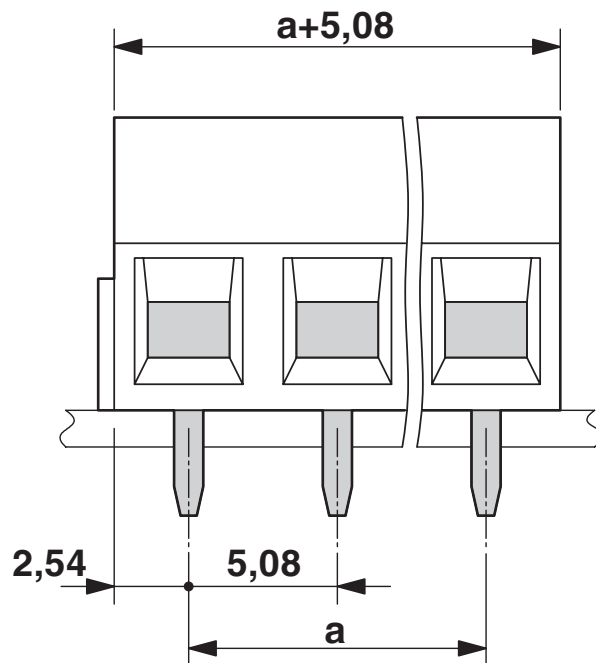
Målskisse
