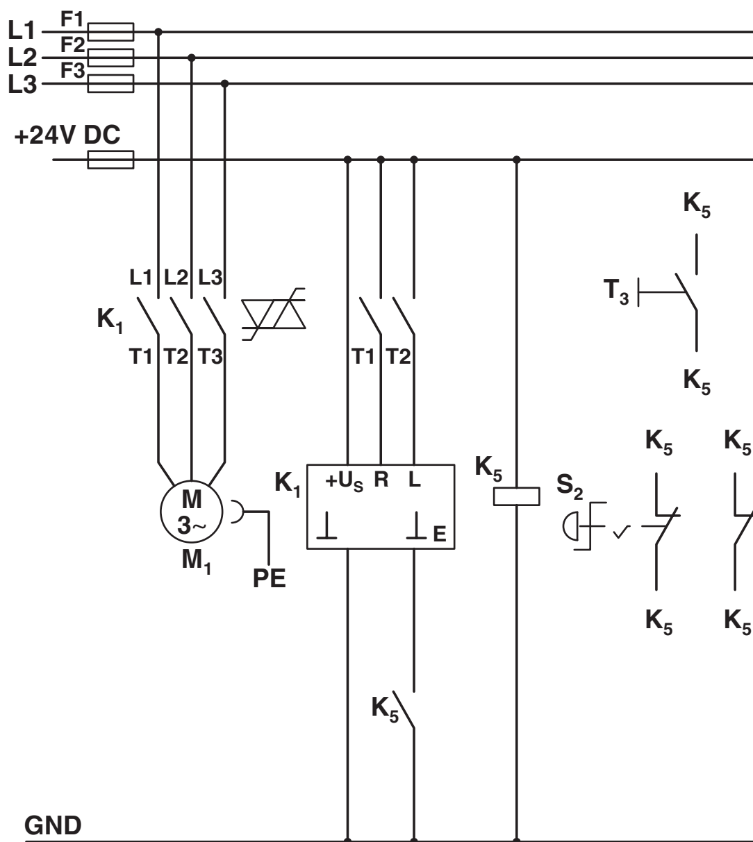
Koblingsskjema
