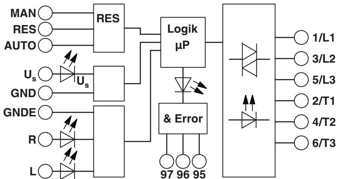
Blokkskjema
