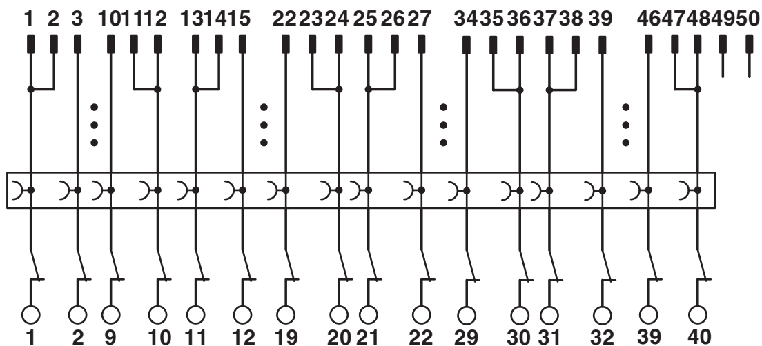
Koblingsskjema
