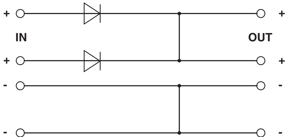
Blokkskjema
