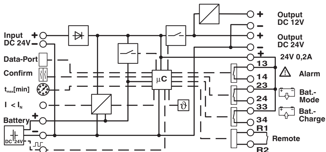
Blokkskjema
