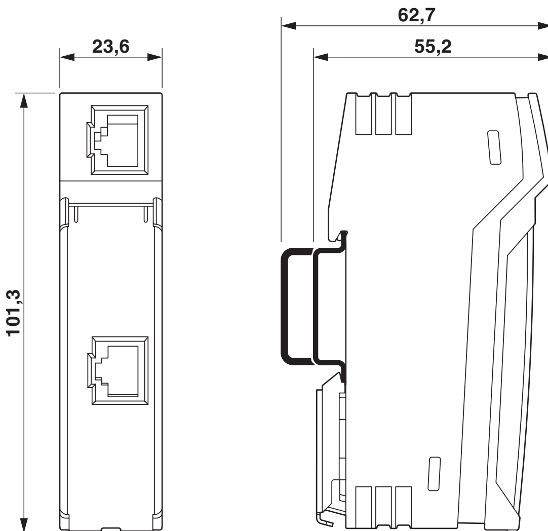
Målskisse
