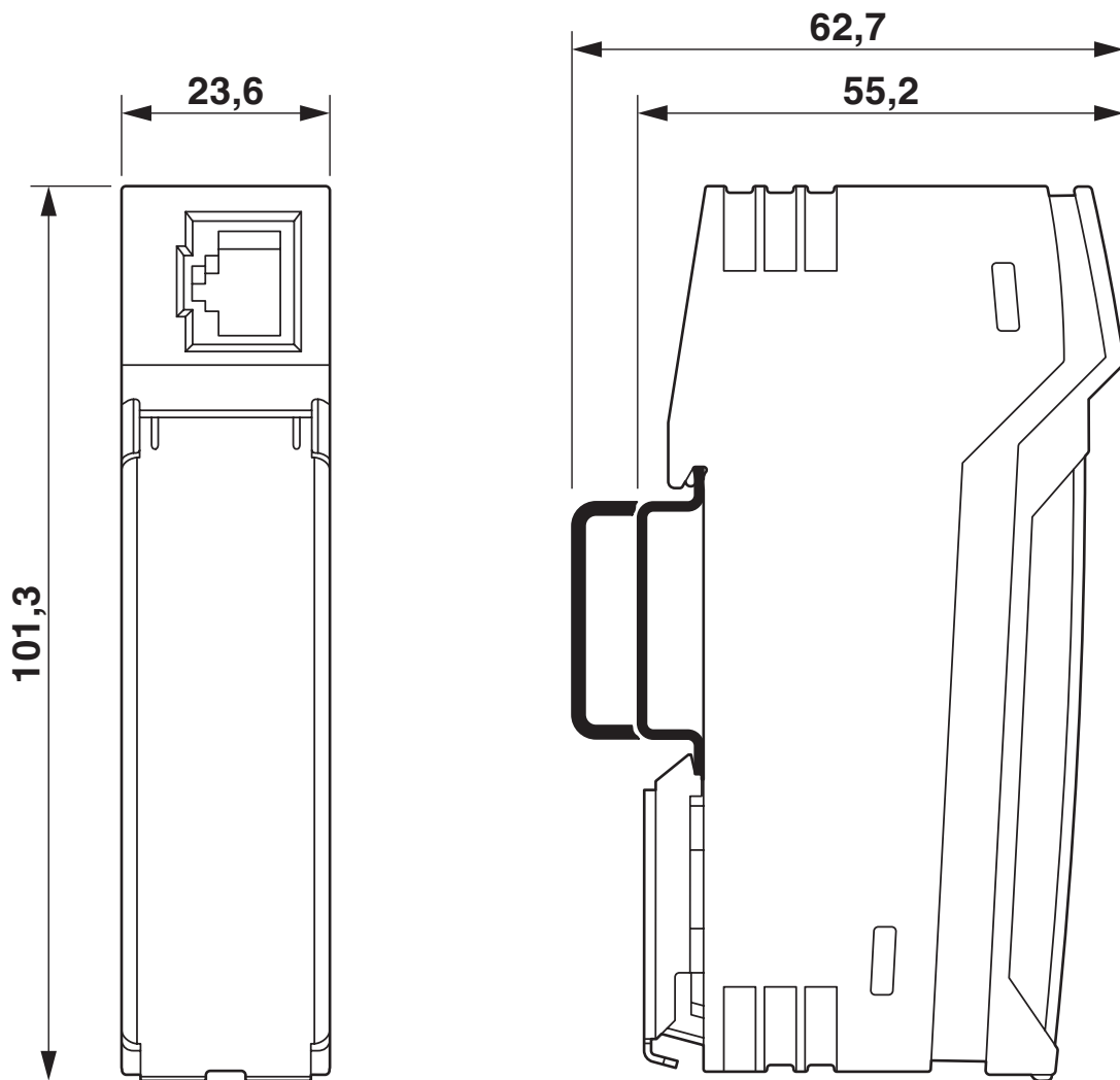
Målskisse
