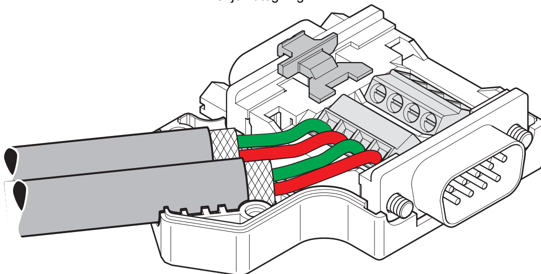
Kabeltilføring på venstre side
