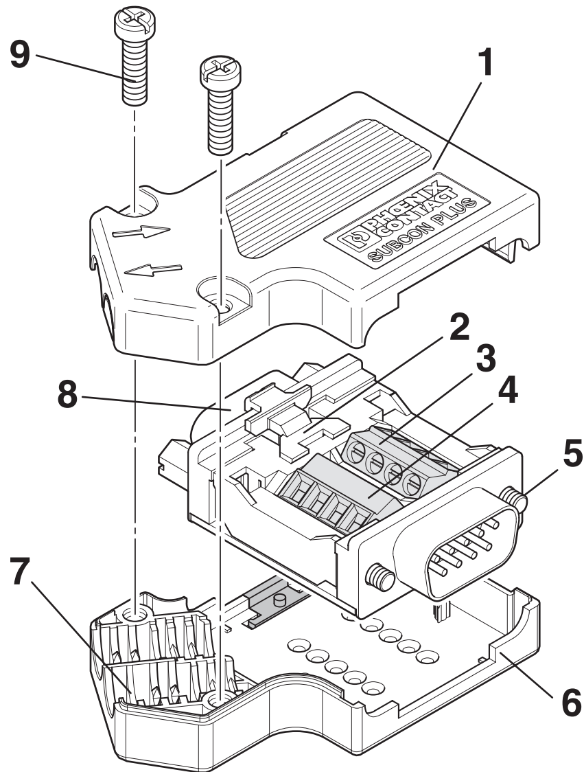
Skjemategning
