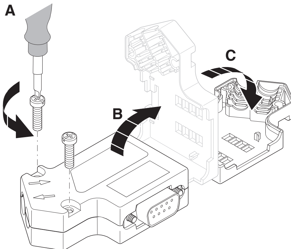
Skjemategning
