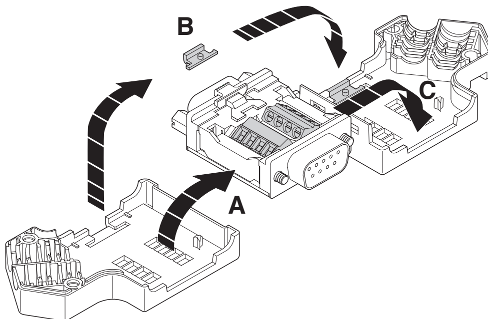
Skjemategning
