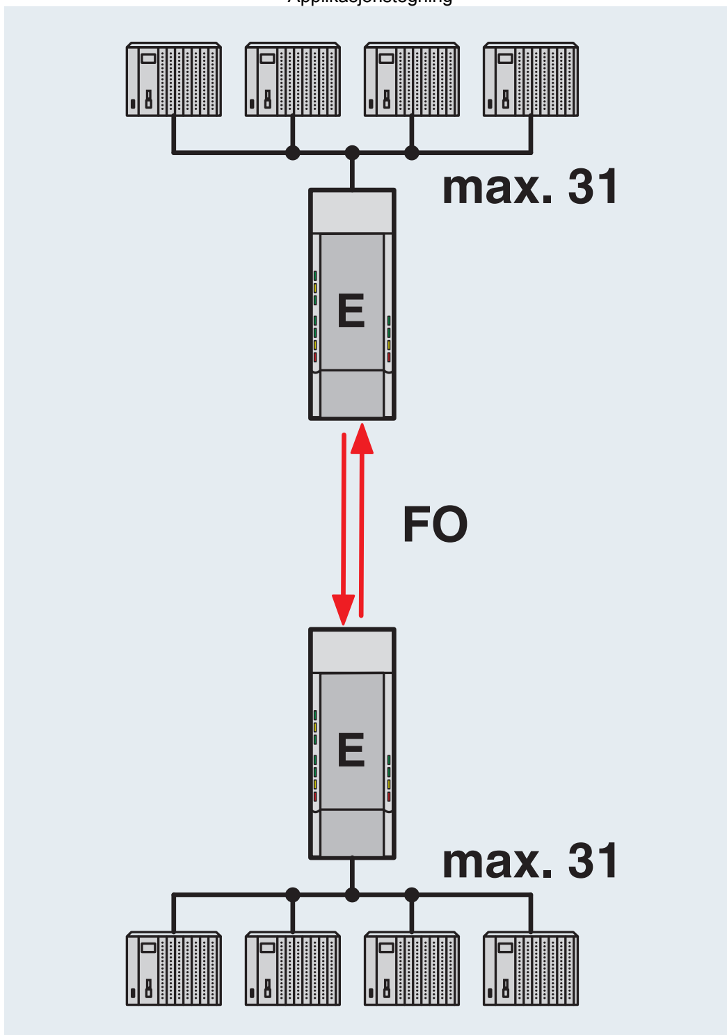
Applikasjonstegning
