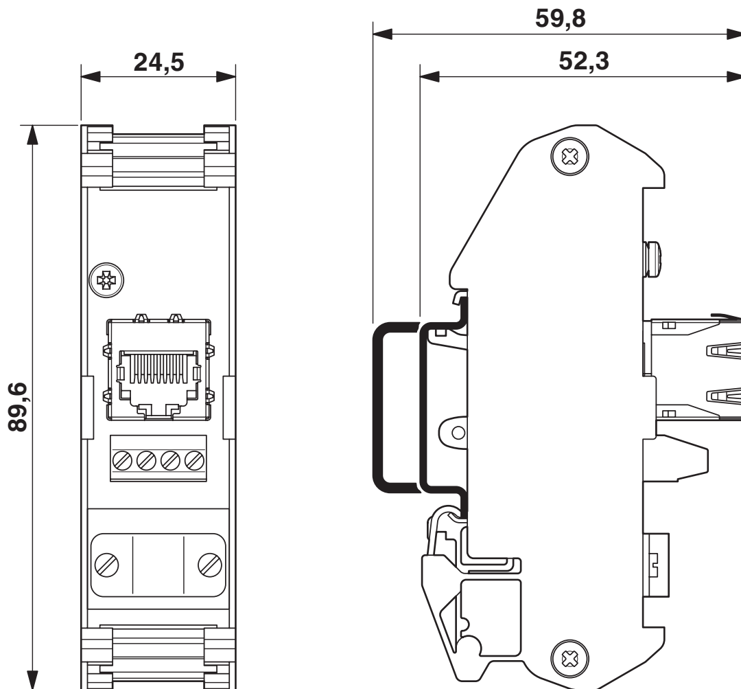
Målskisse
