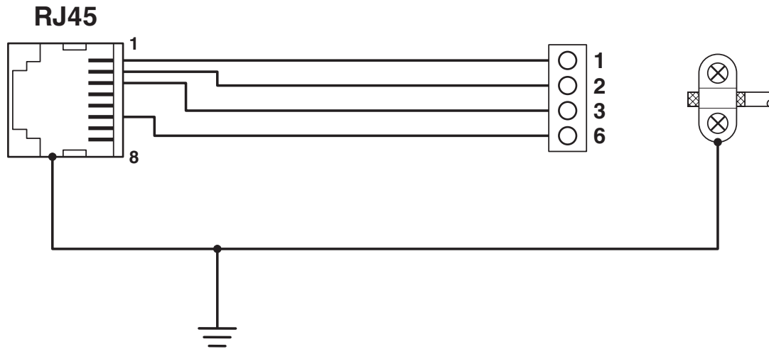
Koblingsskjema
