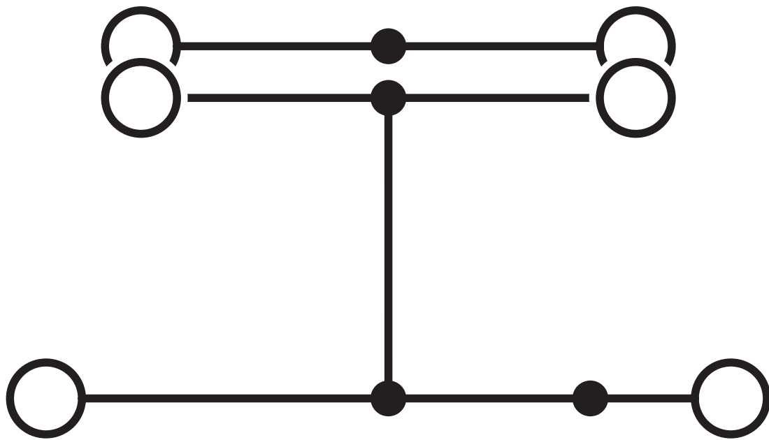
Koblingsskjema
