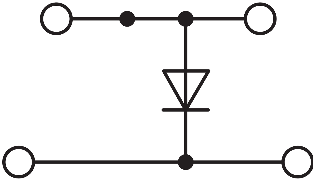
Koblingsskjema
