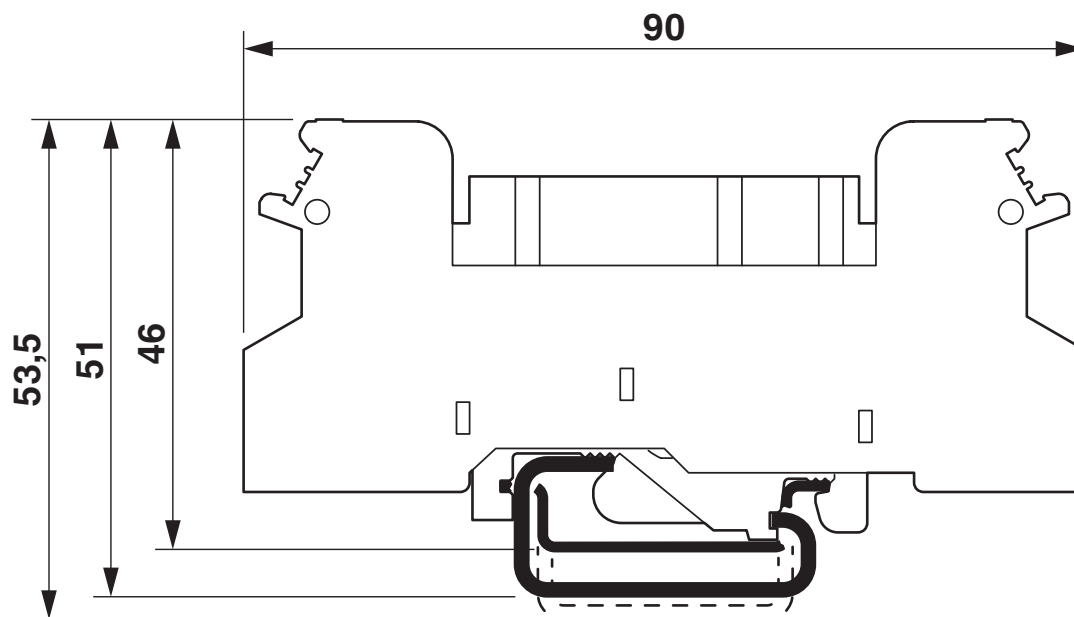
Målskisse
