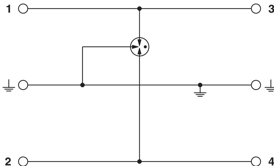
Koblingsskjema
