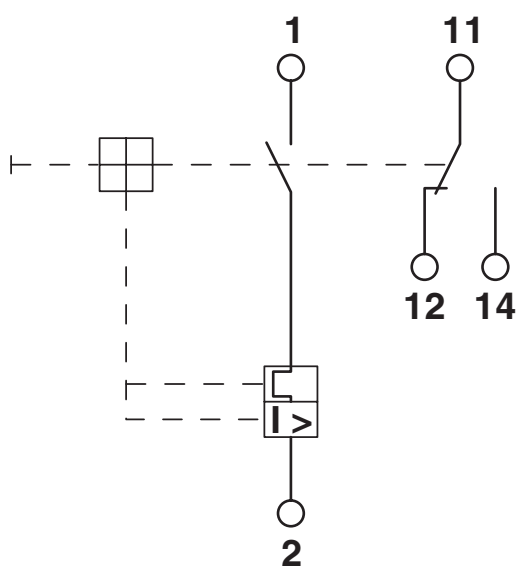
Koblingsskjema
