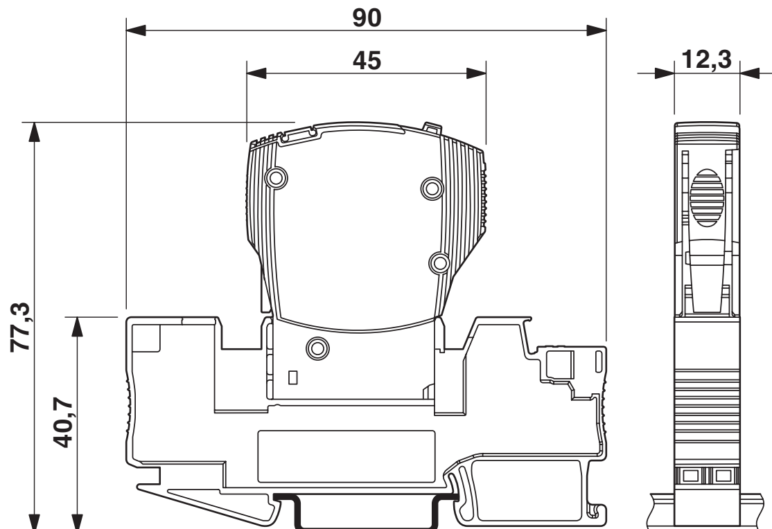
Målskisse
